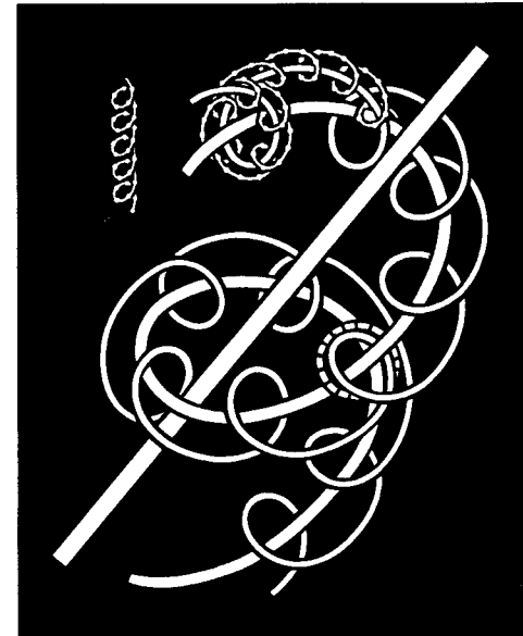
THE SPIRILLAE.
